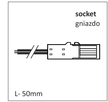
LED cable with MINI socket / black przewód LED MINI 1xG / czarny 2x0,35; L-50
