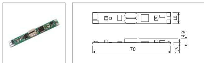
LED 1 channel basic receiver moduł sterujący LED podstawowy 1 kanałowy 12V-24V/72W
