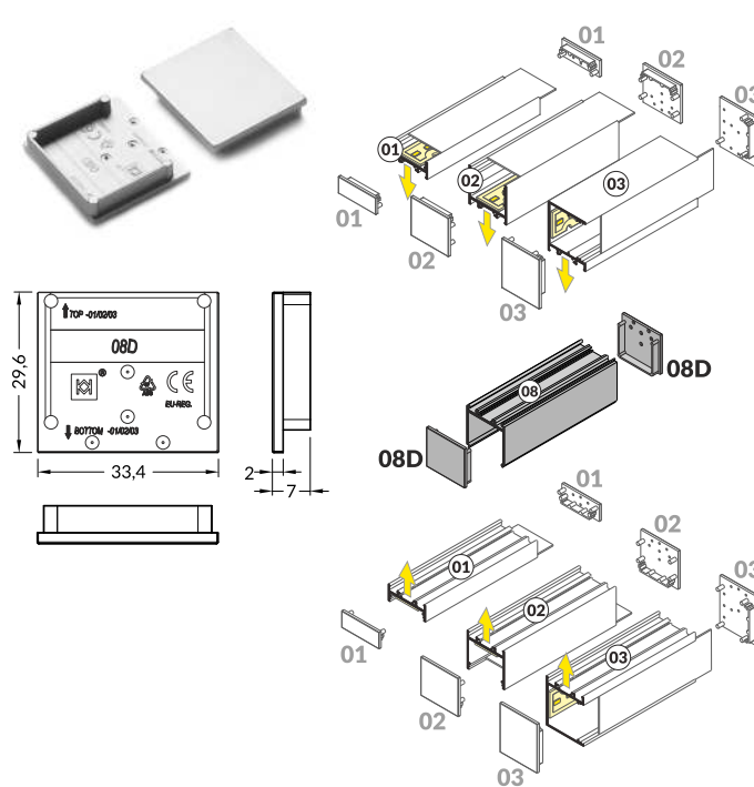
VARIO30-08D ending / zaślepka VARIO30-08D
