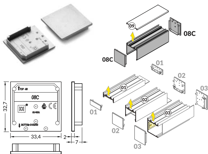
VARIO30-08C ending / zaślepka VARIO30-08C
