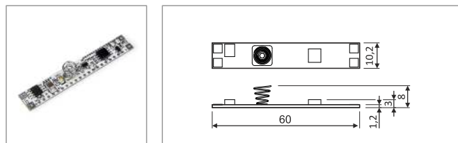
touch LED INSIDE dimmable switch włącznik dotykowy ściemniający LED INSIDE 12-24V/36W
