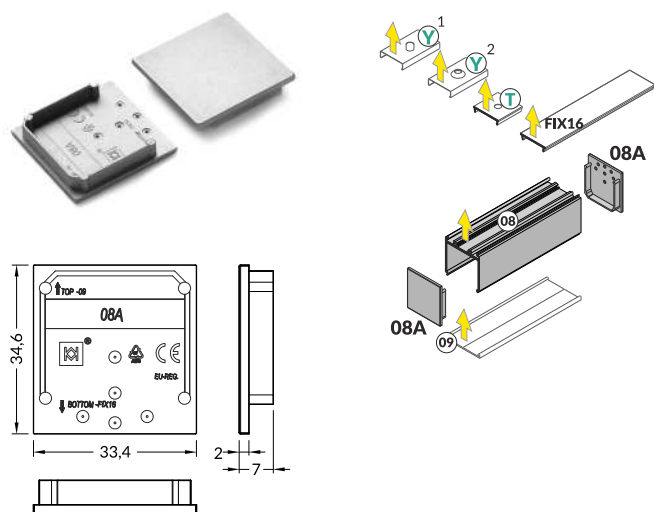
VARIO30-08A ending / zaślepka VARIO30-08A
