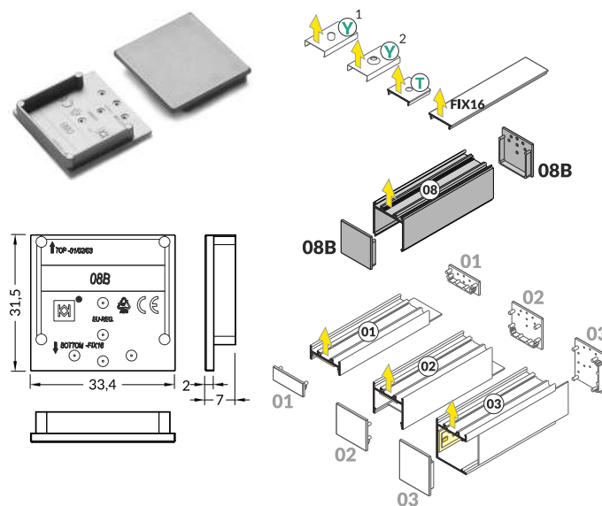
VARIO30-08B ending / zaślepka VARIO30-08B
