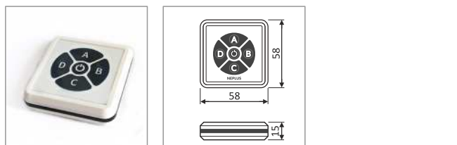
LED 4 channel basic remote controller pilot sterujący LED podstawowy 4 kanałowy
