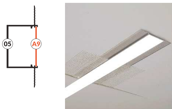
variant 05 - recessed 05-A9 spackle mounting wariant 05 - wpustowy 05-A9 do szpachlowania
