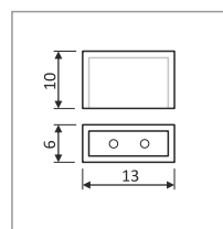
ending for silicone housing for 8 mm LED strip zaślepka do osłony silikonowej do taśmy LED 8 mm
