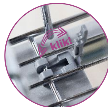
D - blokady dwustronne kosza - bez użycia narzędzi
