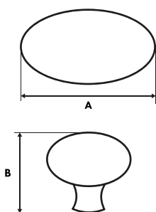
WYMIARY GAŁKI MEBLOWEJ
