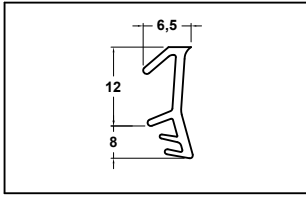
PERFIL EN REPOSO PROFIL USZCZELKI
