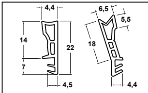
PERFIL EN REPOSO PROFIL USZCZELKI
